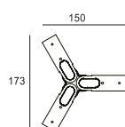
LM-XL015-Y Connecteur EN Y
