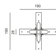
LMO15-X Connecteur en forme X
