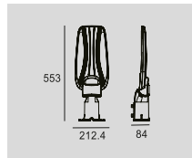
LMR02-150W
