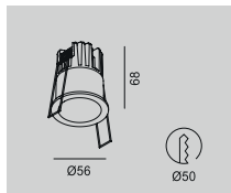
LM8275
