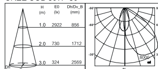
CREE COB 50W-30°
